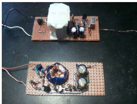
Deux prototypes pour deux principes différents de génération de la HT.
