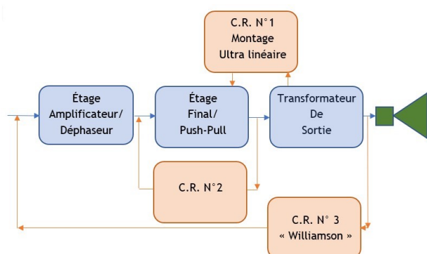
Synoptique des trois types de contre-réaction adoptés
