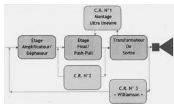
Figure 3 : Synoptique de la contre-réaction de l'Amplifi MKII
