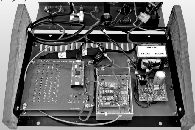
MODULATEUR AM8 COFFRET DU PROTOTYPE
