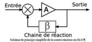
Figure 2 : Schéma de principe simplifié de la contre-réaction en Hi-Fi
